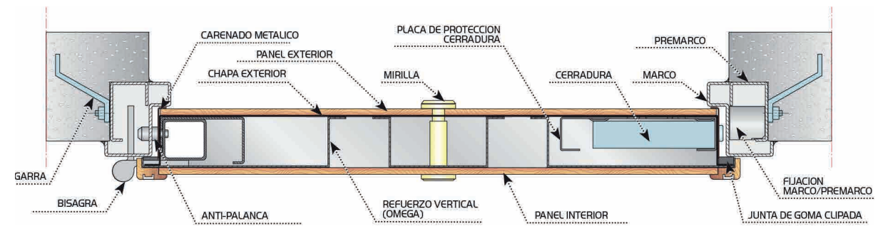
Sección horizontal
