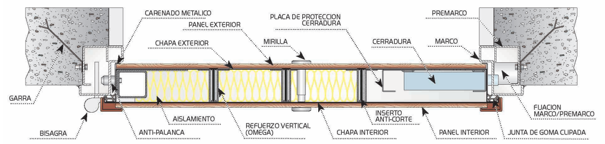
Sección horizontal
