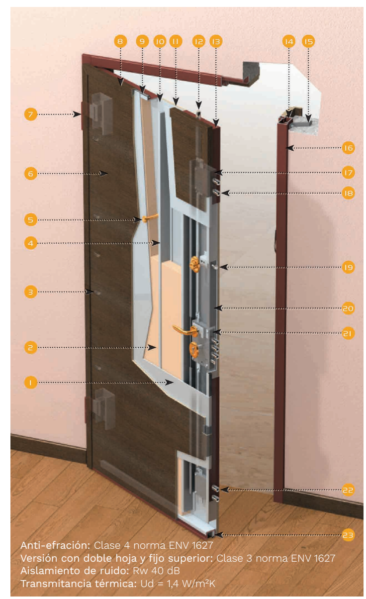
Esquema cerradura
