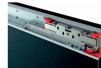
Sistema corredera invisible parte superior
