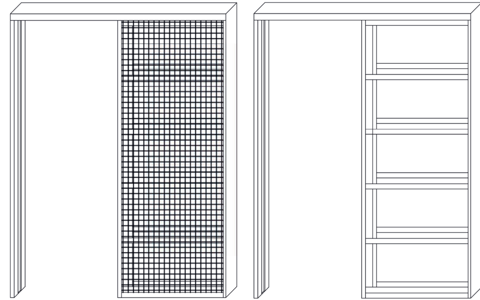
Armazón corredero montaje para revoque
