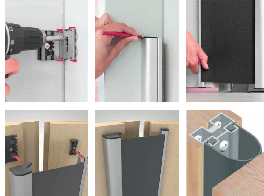
Sistema antipillados FINGERPRO ROLL
