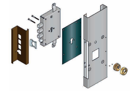
Esquema cerradura
