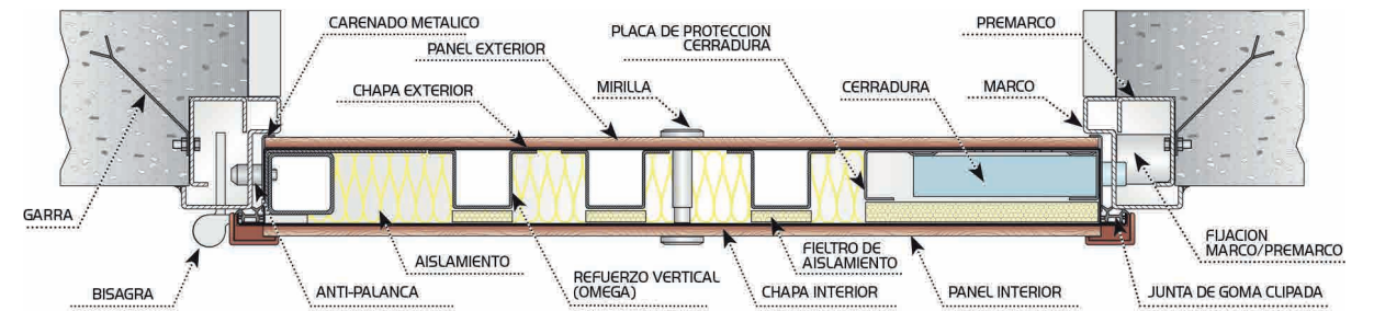
Sección horizontal
